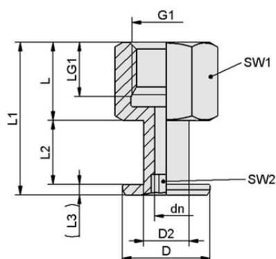
Конструктивные данные SA-NIP N015 G1/4-IG DN600
