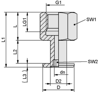
Tasarım verileri SA-NIP N013 G1/4-IG DN350
