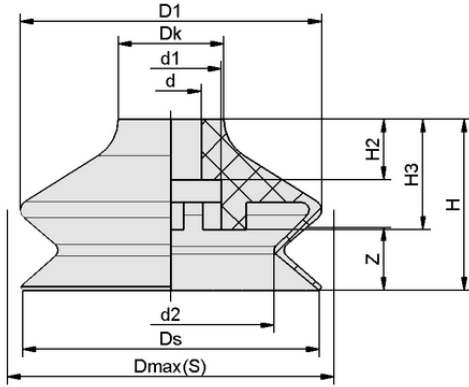
Tasarım verileri FGA 85 VU1-72 N015
