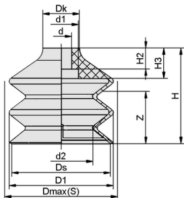
Données de construction FG 85 VU1-72 N015
