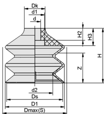
Конструктивные данные FG 85 VU1-72 N015
