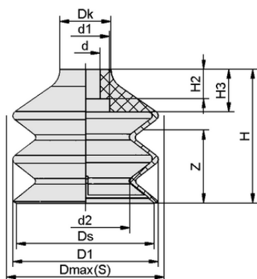
Конструктивные данные FG 30 VU1-72 N013
