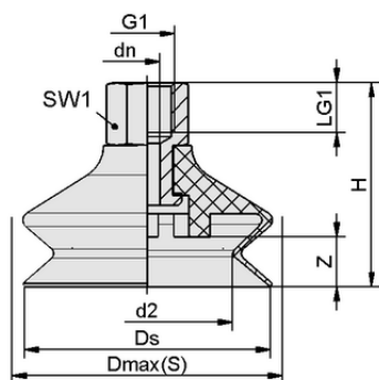
Конструктивные данные FSGA 60 VU1-72 G1/4-IG ON
