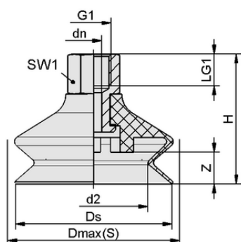
デザインデータ FSGA 60 VU1-72 G1/4-IG ON
