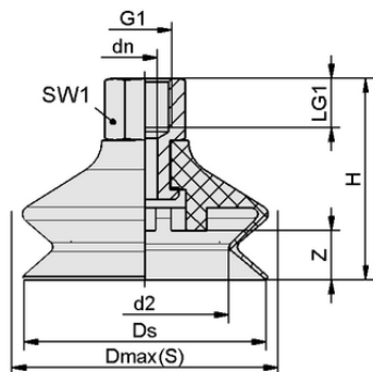
デザインデータ FSGA 30 VU1-72 G1/4-IG
