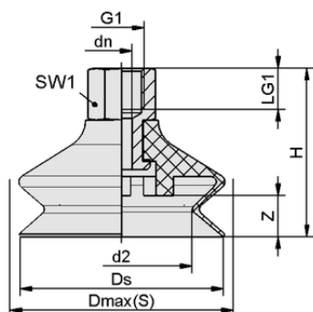
Конструктивные данные FSGA 30 VU1-72 G1/4-IG
