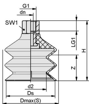
デザインデータ FSG 85 VU1-72 G1/4-IG ON
