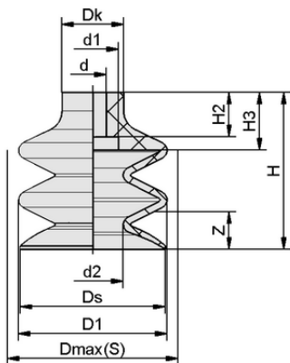
Datos de diseño FG 62 NBR-55 N018
