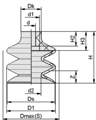
デザインデータ FG 42 NBR-55 N018
