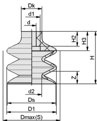
Données de construction FG 32 NBR-55 N018
