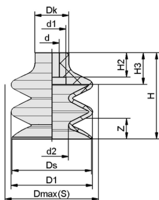
Конструктивные данные FG 32 NBR-55 N018
