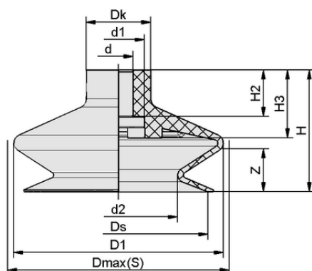
Конструктивные данные FGA 78 NBR-55 N019
