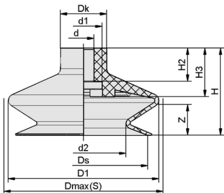
Datos de diseño FGA 53 NBR-55 N018
