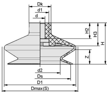
Datos de diseño FGA 33 NBR-55 N018
