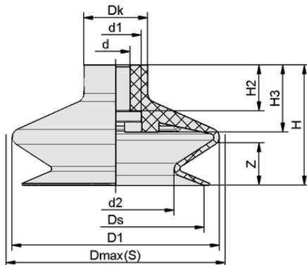
Dati di costruzione FGA 43 SI-55 N018
