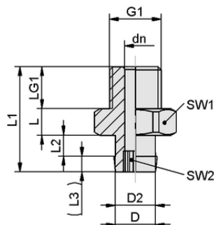
Конструктивные данные SA-NIP N016 M5-AG DN250
