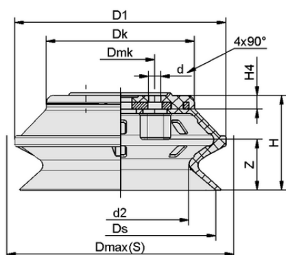
デザインデータ FGA 110 SI-55 N010
