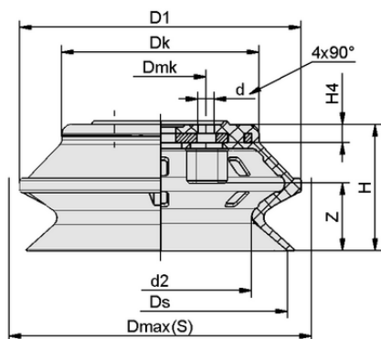
Конструктивные данные FGA 110 SI-55 N010
