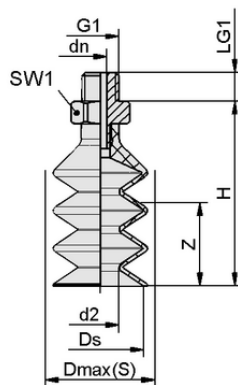
デザインデータ FSGB 25 SI-55 G1/8-AG
