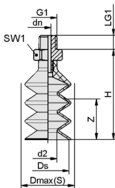
デザインデータ FSGB 25 NBR-55 G1/8-AG
