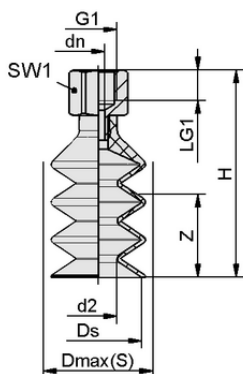
Datos de diseño FSGB 25 SI-55 G1/8-IG
