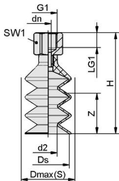
Конструктивные данные FSGB 25 SI-55 G1/8-IG
