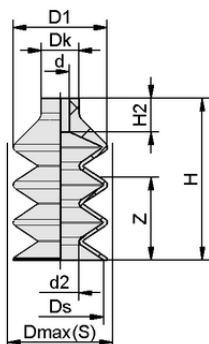
Конструктивные данные FGB 25 NBR-55 N049
