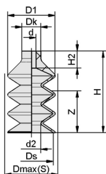
デザインデータ FGB 25 NBR-55 N049
