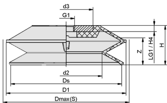
Конструктивные данные FSGPL 250 NBR-55 G1/2-IG
