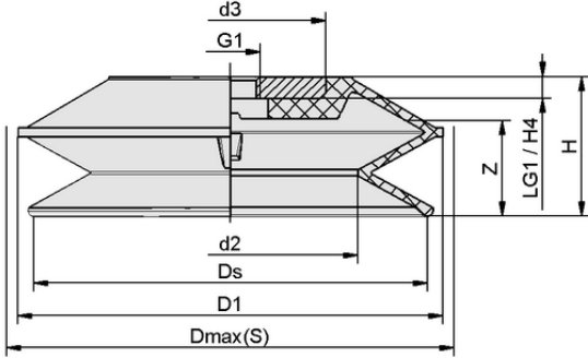
Tasarım verileri FSGPL 150 NBR-55 G1/2-IG
