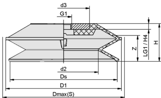
Dati di costruzione FSGPL 150 NBR-55 G1/2-IG
