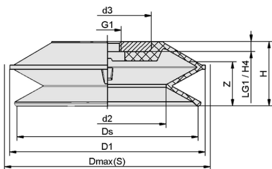
Конструктивные данные FSGPL 150 NBR-55 G1/2-IG
