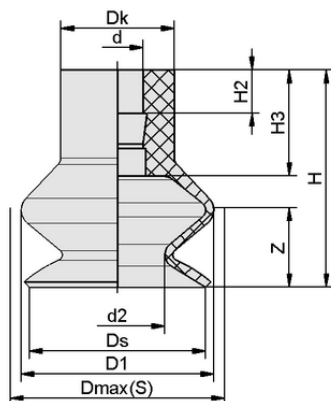
Конструктивные данные FGA 11 SI-55 N016
