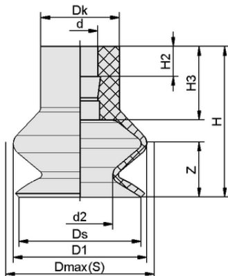
Dati di costruzione FGA 22 NBR-55 N016
