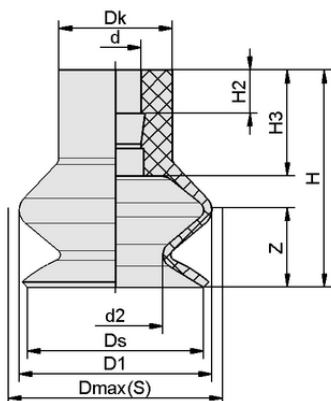
Datos de diseño FGA 16 NBR-55 N016
