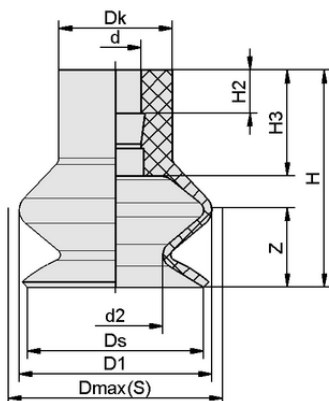
Datos de diseño FGA 11 NBR-55 N016
