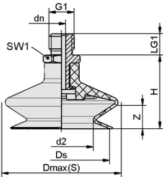
Tasarım verileri FSGA 22 SI-55 G1/8-AG
