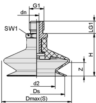
Datos de diseño FSGA 22 SI-55 G1/8-AG
