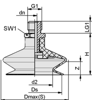
Конструктивные данные FSGA 11 SI-55 M5-AG
