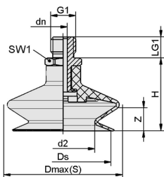
デザインデータ FSGA 16 NBR-55 M5-AG
