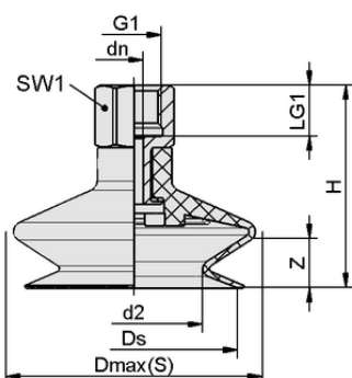
Dati di costruzione FSGA 22 SI-55 G1/8-IG
