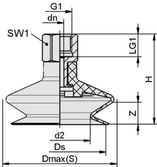
Tasarım verileri FSGA 16 NBR-55 G1/8-IG
