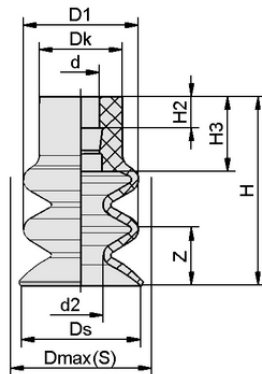
Données de construction FG 20 SI-55 N016
