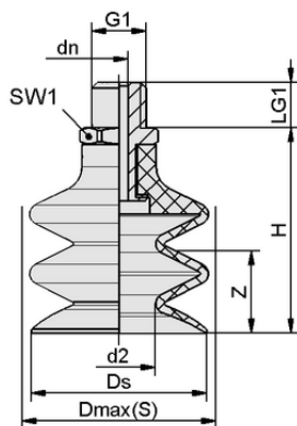
Dati di costruzione FSG 18 SI-55 M5-AG
