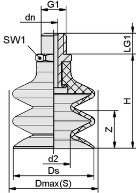
Tasarım verileri FSG 14 SI-55 M5-AG
