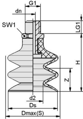
Tasarım verileri FSG 14 SI-55 G1/8-AG
