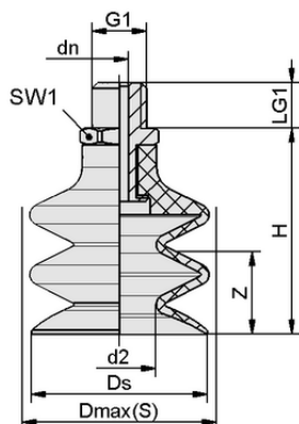
Конструктивные данные FSG 20 NBR-55 G1/8-AG
