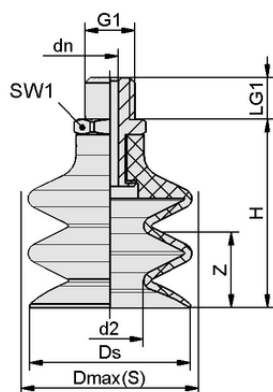
デザインデータ FSG 14 NBR-55 G1/8-AG
