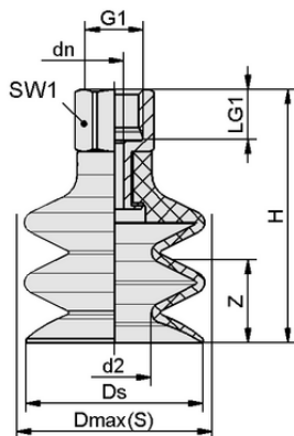
Dati di costruzione FSG 14 SI-55 G1/8-IG
