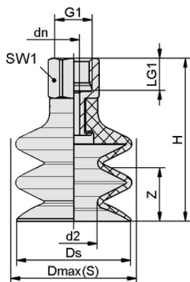
デザインデータ FSG 18 NBR-55 G1/8-IG
